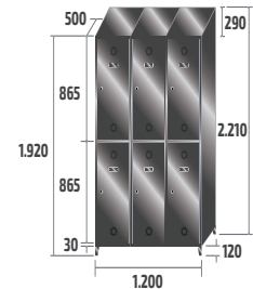
SV-40/3 INOX COD: 84903 82kg · 1,14m 3
