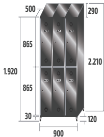
SV-30/3 INOX COD: 83903 67kg · 0,99m 3
