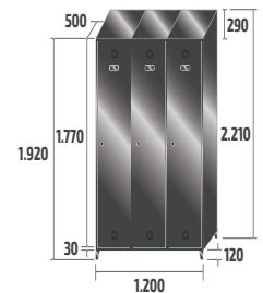
SV-40/3 INOX COD: 84903 82kg · 1,14m 3
