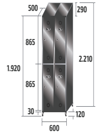
SV-30/2 INOX COD: 83902 49kg · 0,69m 3
