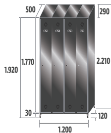
SV-30/4 INOX COD: 83904 85kg · 1,31m 3
