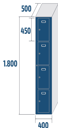
STV4-40/1 COD: 44841 28kg · 0,29m 3
