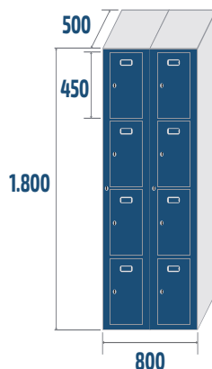
STV4-40/2 COD: 44842 50kg · 0,57m 3
