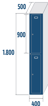
STV2-40/1 COD: 44821 25kg · 0,29m 3
