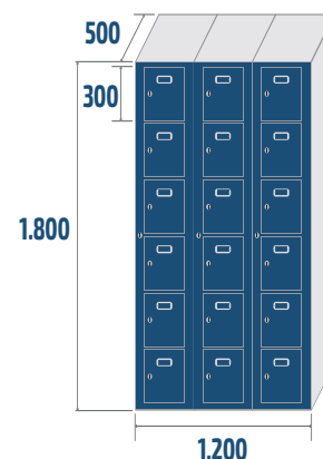
STV6-40/3 COD: 44863 78kg · 1,08m 3
