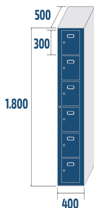
STV6-40/1 COD: 44861 30kg · 0,29m 3
