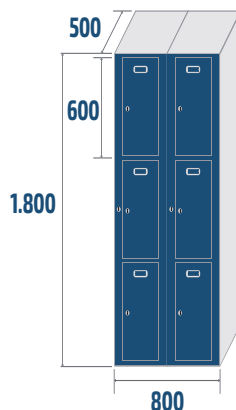
STV3-40/2 COD: 44832 45,8kg · 0,57m 3
