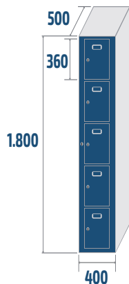
STV5-40/1 COD: 44851 29kg · 0,29m 3
