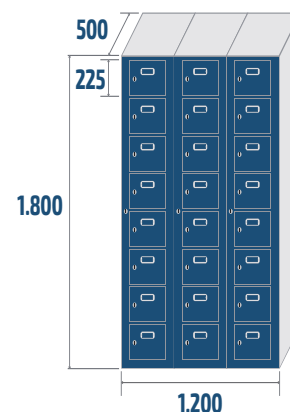
STV8-40/3 COD: 44883 81kg · 1,08m 3
