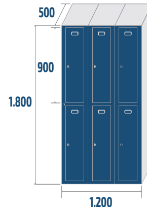
STV2-40/3 COD: 44823 65kg · 1,08m 3
