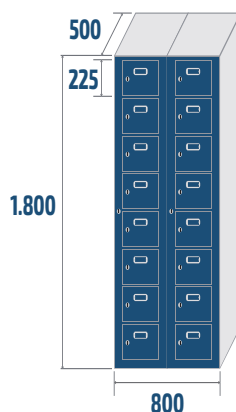
STV8-40/2 COD: 44882 56kg · 0,57m 3
