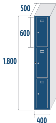
STV3-40/1 COD: 44831 25,9kg · 0,29m 3
