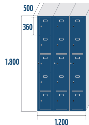
STV5-40/3 COD: 44853 72kg · 1,08m 3
